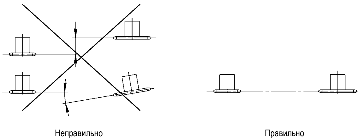
Рис.13 Выравнивание звездочек
