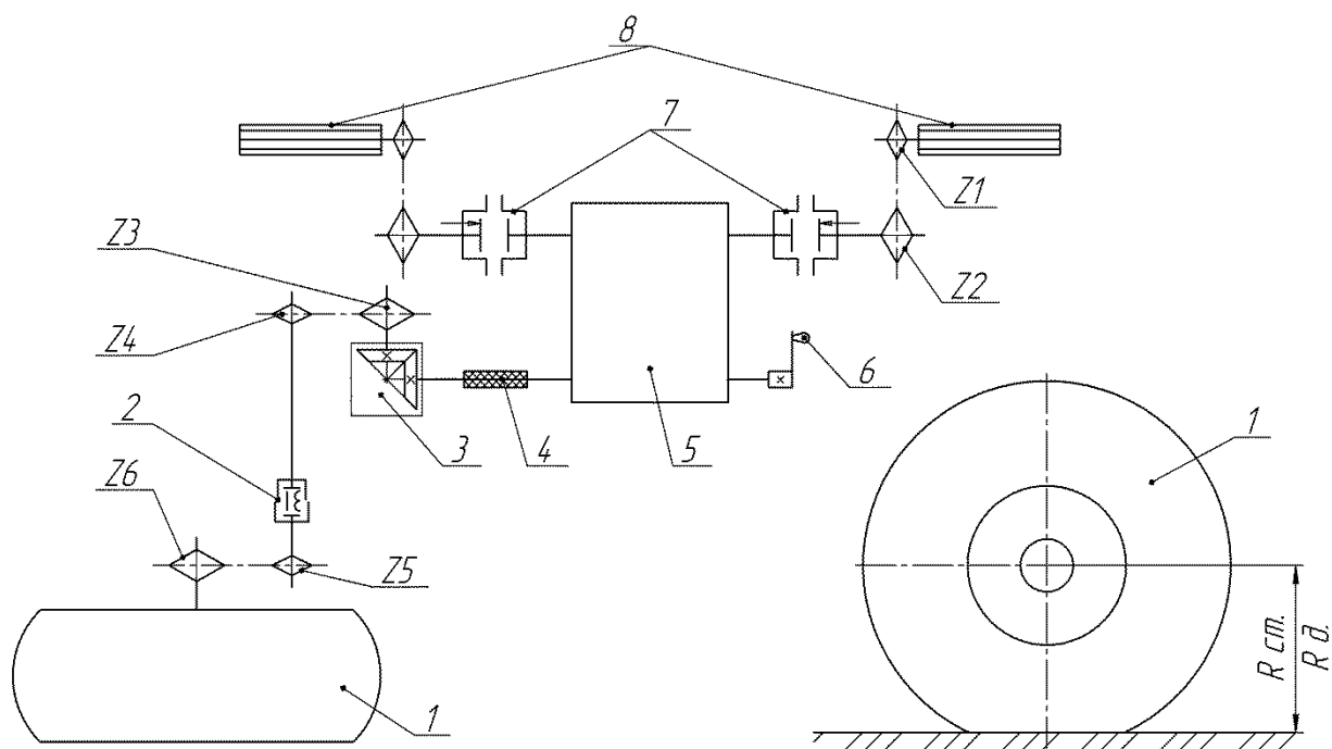
Рис.15 Кинематическая схема
