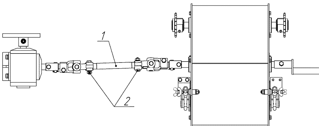
Рис.14 Карданный привод 1 – вал; 2 – болт фиксирующий
